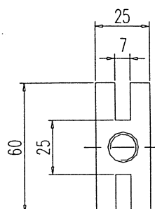
Prüfflansch 60 x 25 x 10 mm
